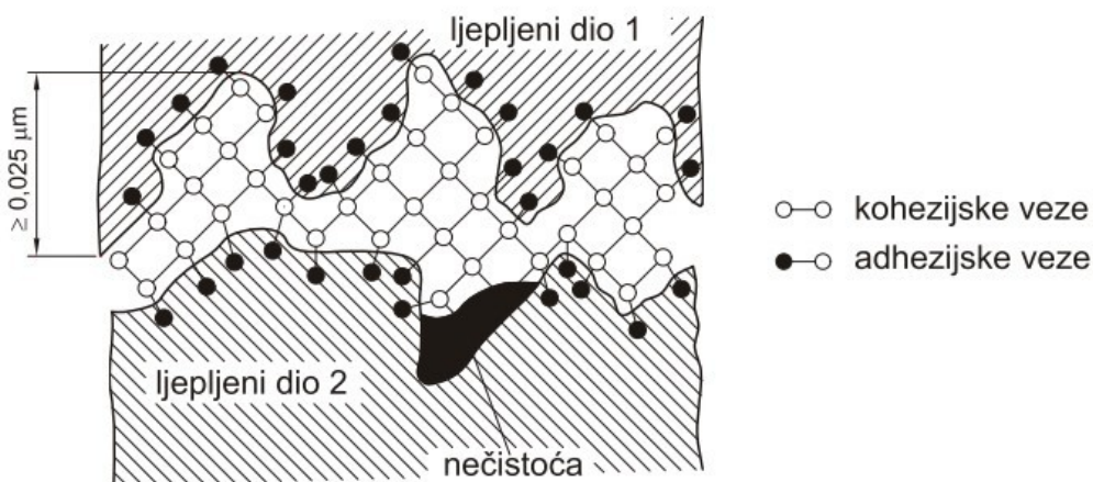
Slika 5.: Fizikalna građa lijepljenog spoja [20]
