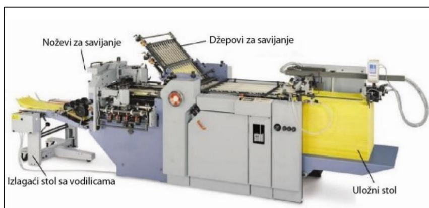
Slika 59. Savijačica
