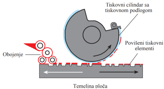
Slika 4.18 a) Princip ploča- valjak, b) Brzotisni knjigotiskarski stroj[12]
