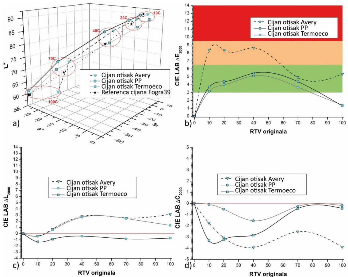
Slika 28. Odstupanje cijan otisaka otisnutih na samoljepljivim materijalima Avery, Polipropilem i Termoecco nastalih na tiskarskom stroju Durst Tau 330 RSC: a) 3D krivulja reprodukcije, b) CIE\ LAB\ \Delta E , c) CIE\ LAB\ \Delta L , d) CIE\ LAB\ \Delta C
