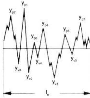
Slika 46 R_z parametar
