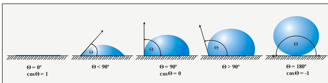
Slika 49 Kontaktni kutovi za različiti stupanj močenja površine
