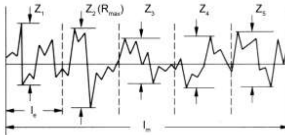
Slika 47 R_{max} parametar
