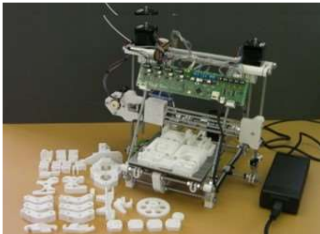
Slika 26 RepRap projekt [17]
