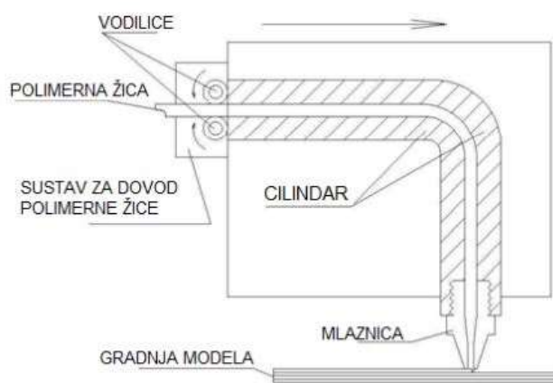
Slika 19 Ekstruder
