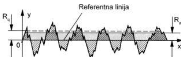
Slika 45 R_a parametar
