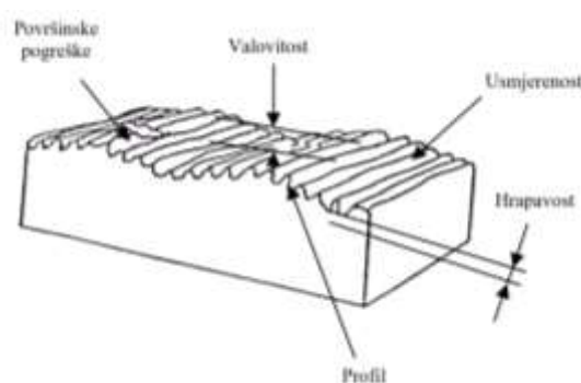
Slika 44 Odstupanja površine
