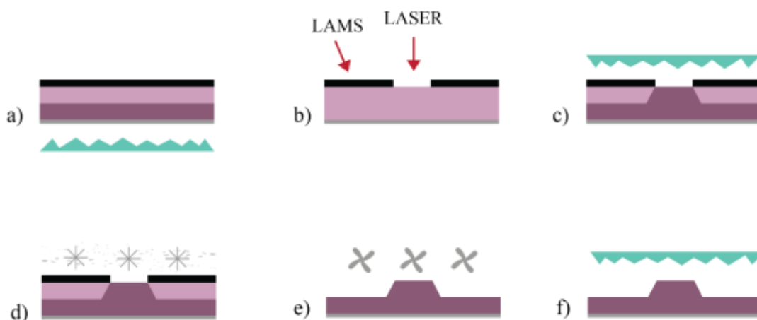
Slika 11 Radne faze izrade tiskovne forme LAMS maskom
