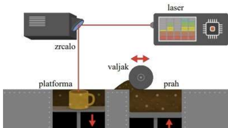
Slika 24 Selektivno lasersko sraščivanje [15]
