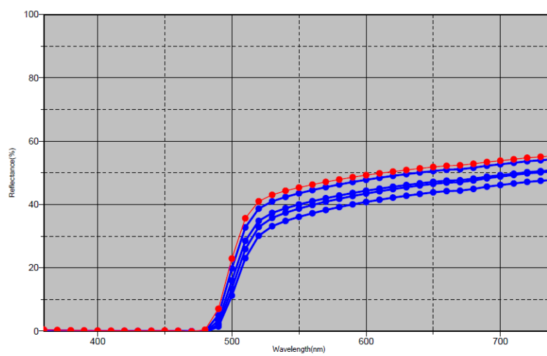
Slika 192 Spektralne krivulje transmissijskih svojstava ispitnih uzoraka s žutim bojilom 1,0 mm - 1,8 mm
