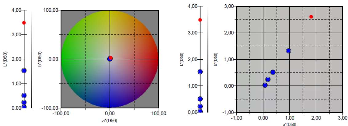
Slika 205 CIELAB prikaz transmisijiskih svojstava ispitnih uzoraka s crnim bojom 1,0 mm – 1,8 mm
