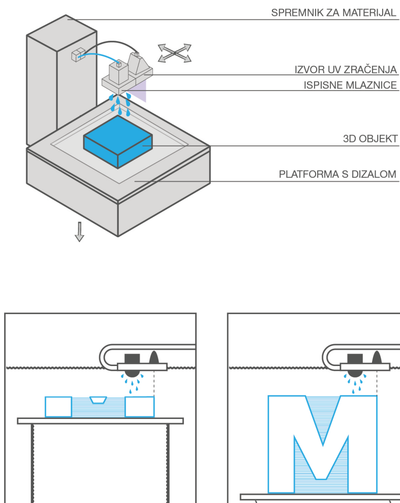
Slika 10 Proces izrade 3D otiska postupkom otiskivanja materijala
