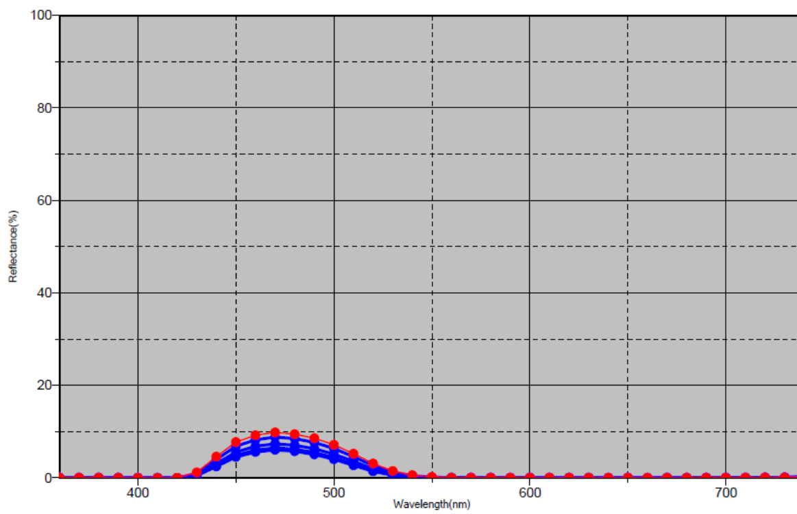
Slika 177 Spektralne krivulje transmisijских svojstava ispitnih uzoraka s cijan bojom 4,0 mm - 4,8 mm
